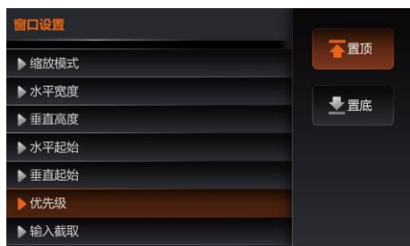
窗口置顶
