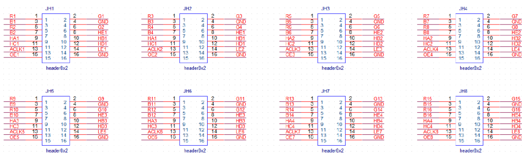
数据接口定义 (以 JH1 为例)
